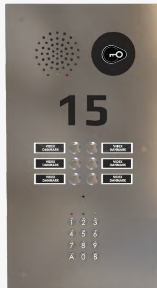
Dørtableau med tryk i dobbeltrække, kodetastatur, ADK og graveret husnummer
